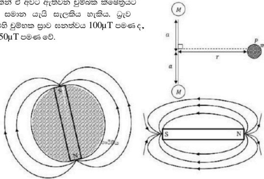
දණ්ඩ චුම්බකය ලෙස ආදේශ කර පෘථිවියේ චුම්බක රේඛාවල ව්‍යාප්තිය දැක්වෙන සටහන
